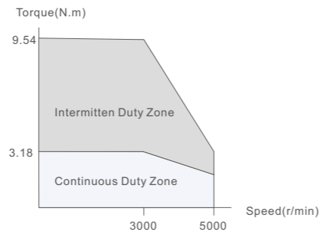
ELM2H - 1000W Motor
