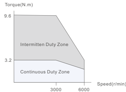
ELM2L - 1000W Motor
